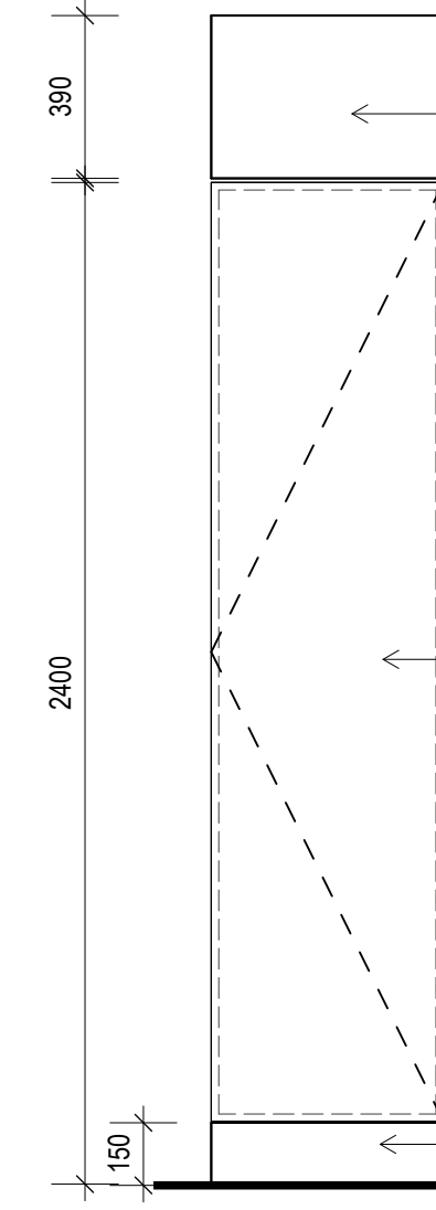
4 ELEVATION JU-04 Scale: 1: 20
