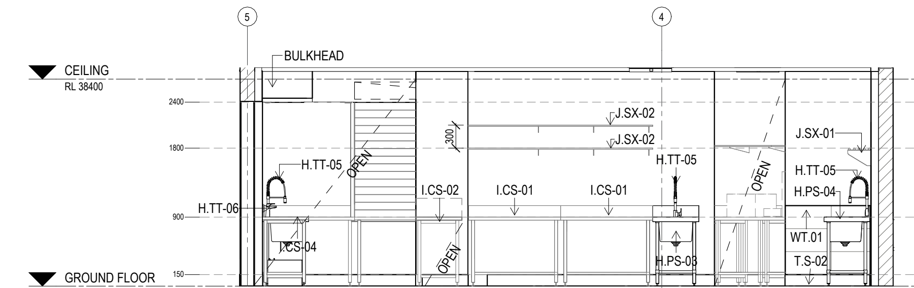
E ELEVATION CANTEEN/KITCHEN Scale: 1: 50
