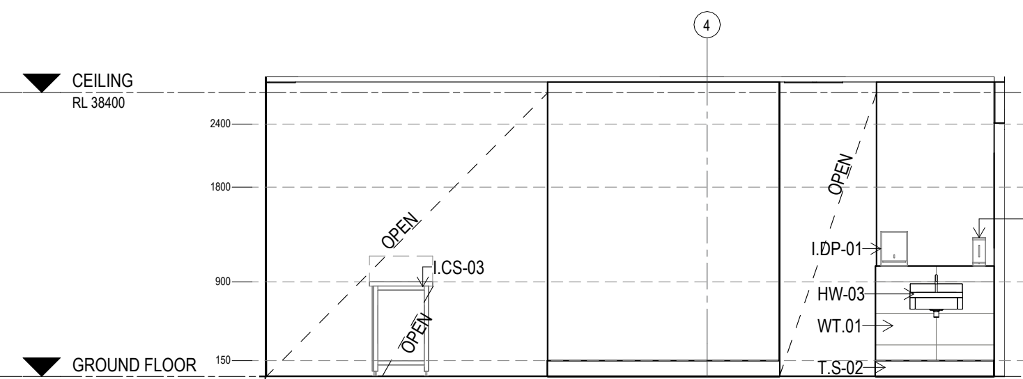
G ELEVATION CANTEEN/KITCHEN Scale: 1: 50
