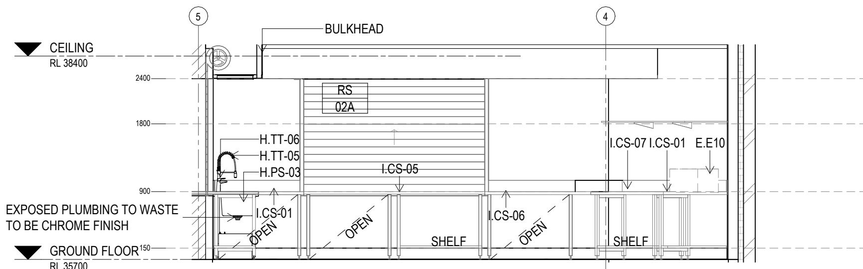
A ELEVATION CANTEEN/KITCHEN Scale: 1: 50
