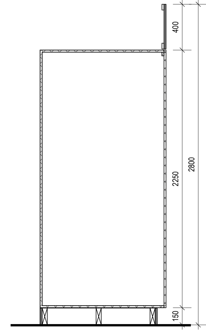
3 DETAIL SECTION JU-04 Scale: 1: 20
